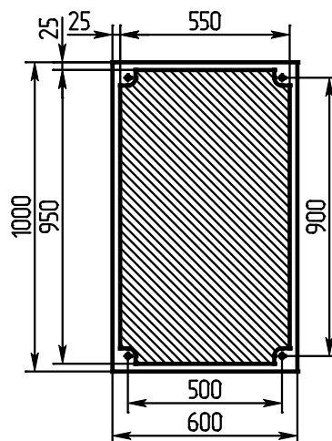
Схема установки шкафа и зона подвода кабеля снизу
